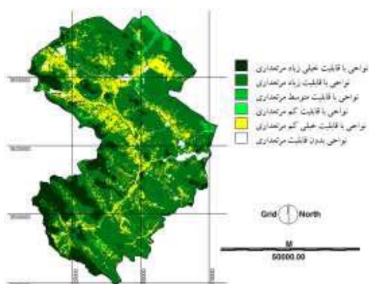
شکل ۴- نقشه قابلیت مرتع داری به روش OWA
