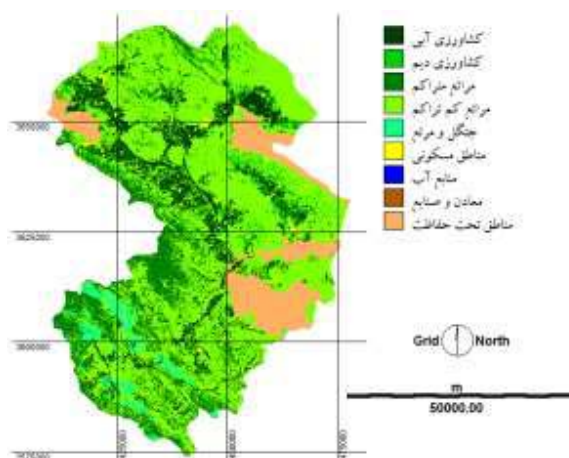
شکل ۲- نقشه کاربری و پوشش اراضی در سال ۱۳۹۴
