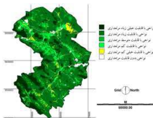
شکل ۳- نقشه قابلیت مرتع داری به روش WLC
